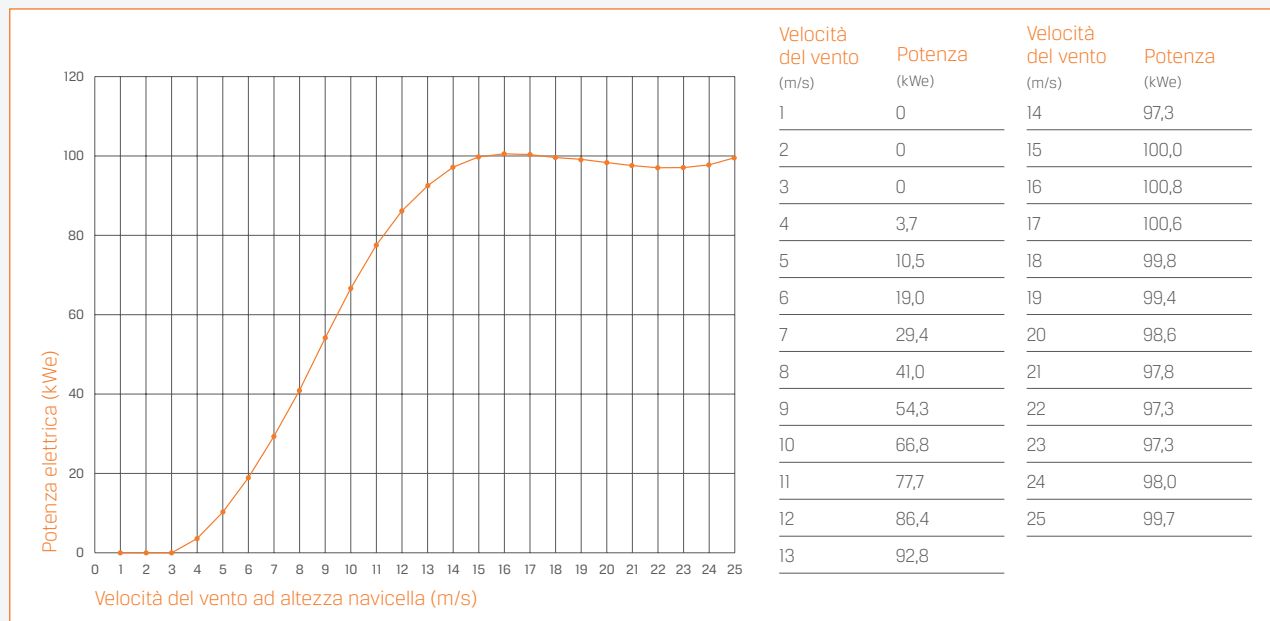
Curva di potenza: rotore di 21 metri Densità standard dell'aria (1.225 kg/m 3 )
