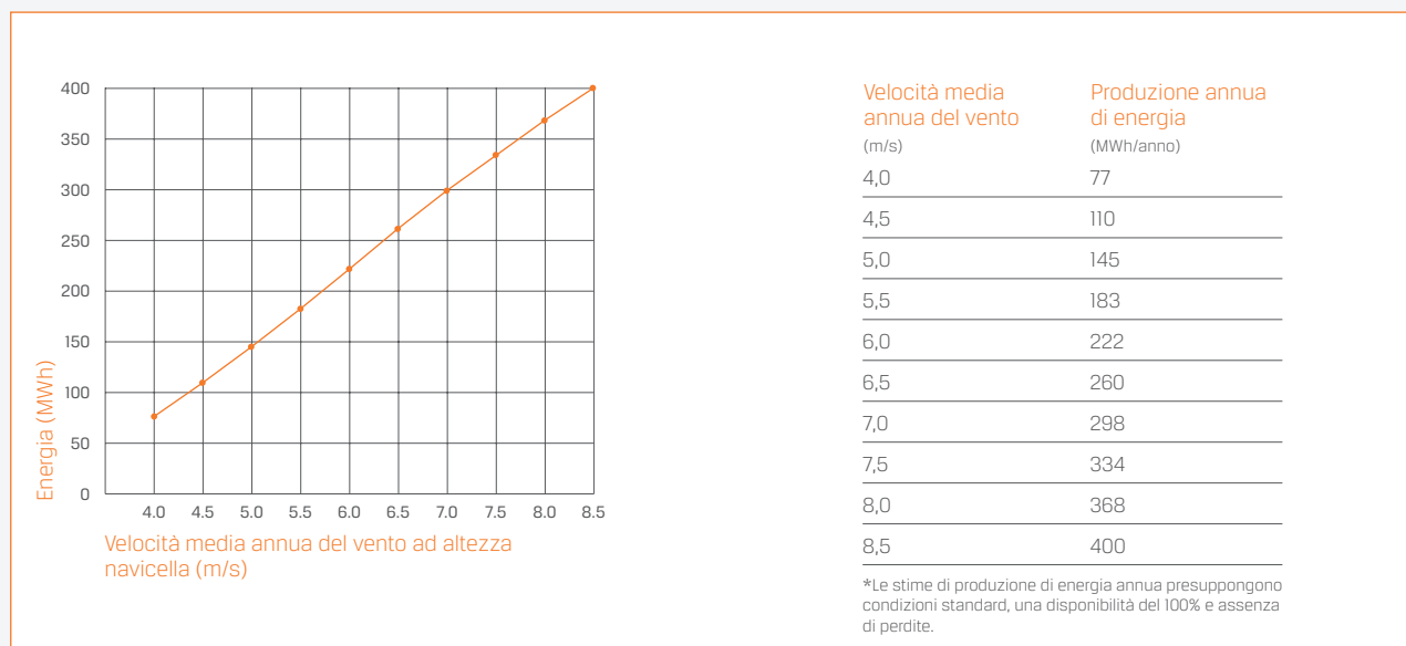
Produzione annua di energia*: rotore di 21 metri Densità standard dell'aria, distribuzione di Rayleigh
